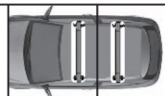
109 mm 135 mm
